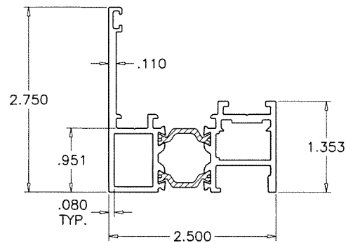
E1 WINDOW FRAME
